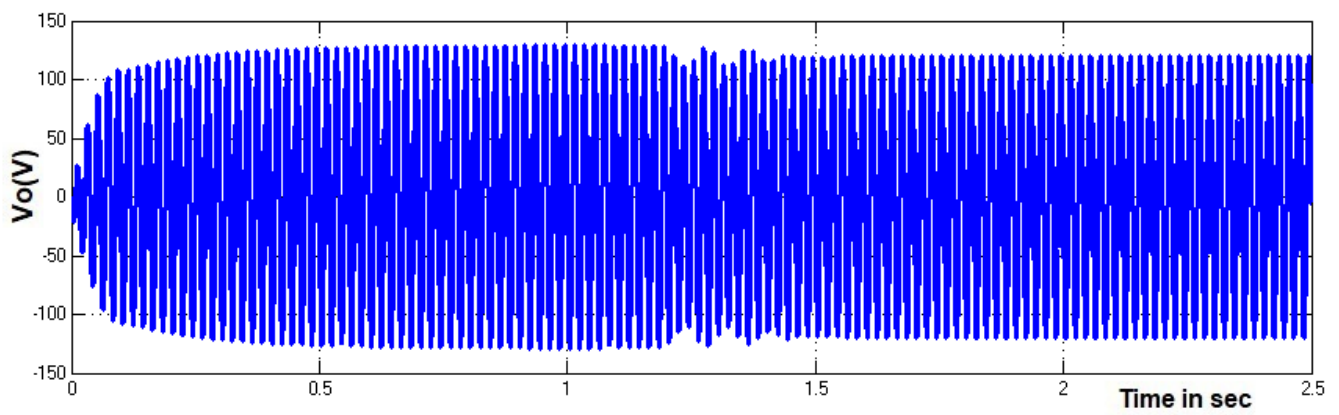
Fig. 30. RL load voltage.
