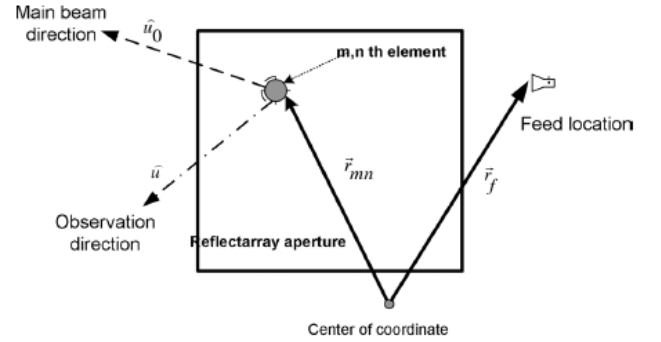
Fig. 5. Reflectarray coordinate system
